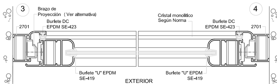
CORTE HORIZONTAL
