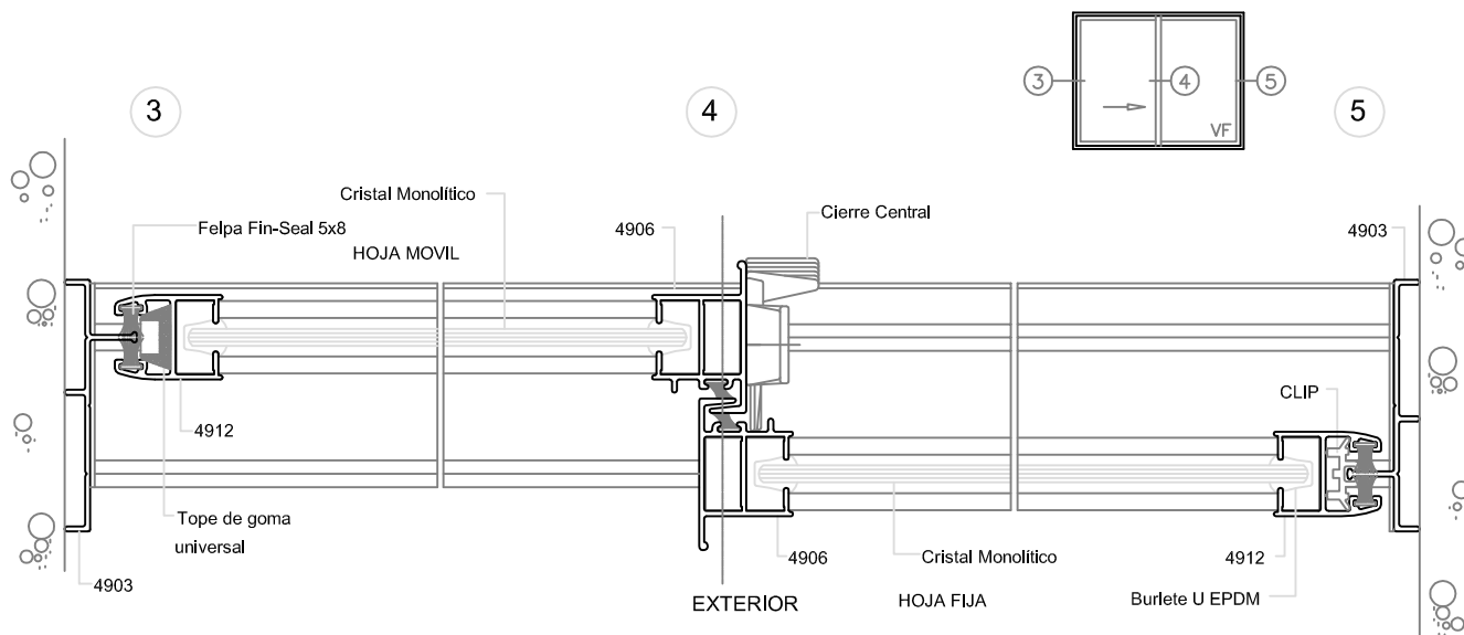
CORTE HORIZONTAL 1 HOJA MOVIL / 1 HOJA FIJA
