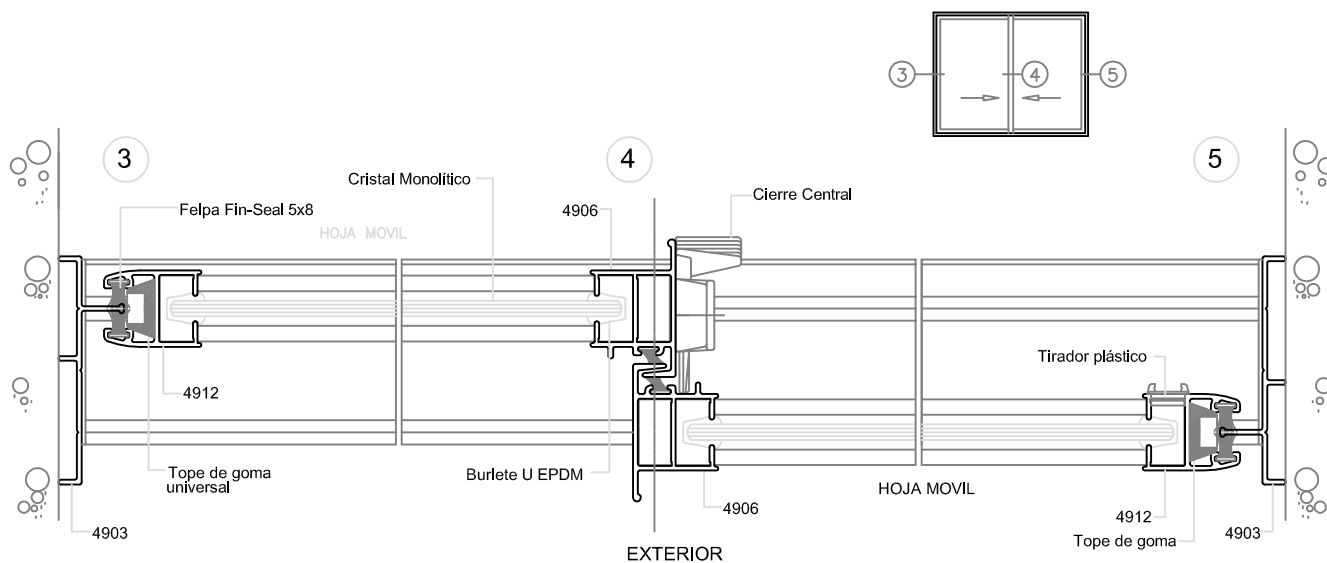
CORTE HORIZONTAL 2 HOJAS MOVILES
