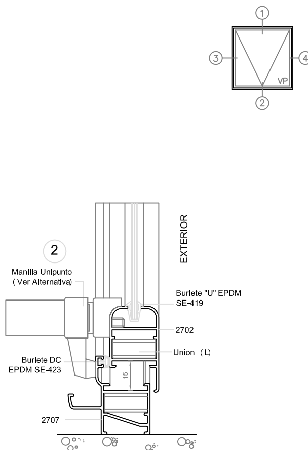
CORTE VERTICAL CAMARA DE AGUA
