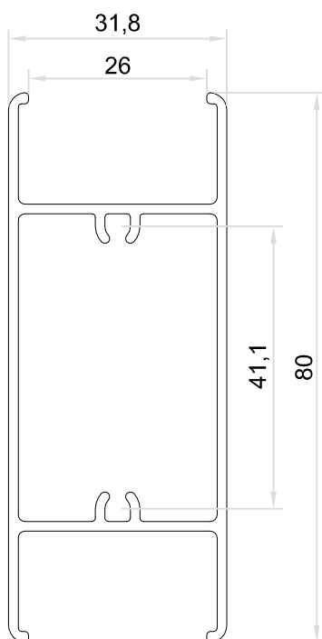
4344 PALILLO DOBLE VIDRIO Peso : 0.906 Kg/M Espesor : 1.4 mm Largo : 6,00 mts
