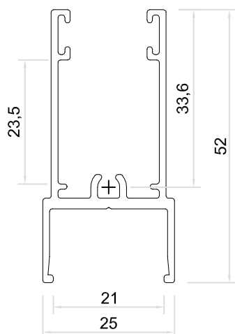
6915 CABEZAL / ZOCALO DVH Peso : 0.569 Kg/M Espesor : 1.3 mm Largo : 6,00 mts
