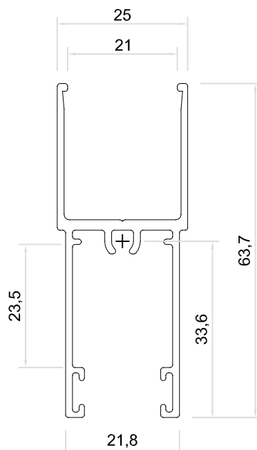
6946 ZOCALO ALTO DVH Peso : 0.654 Kg/M Espesor : 1.3 mm Largo : 6,00 mts
