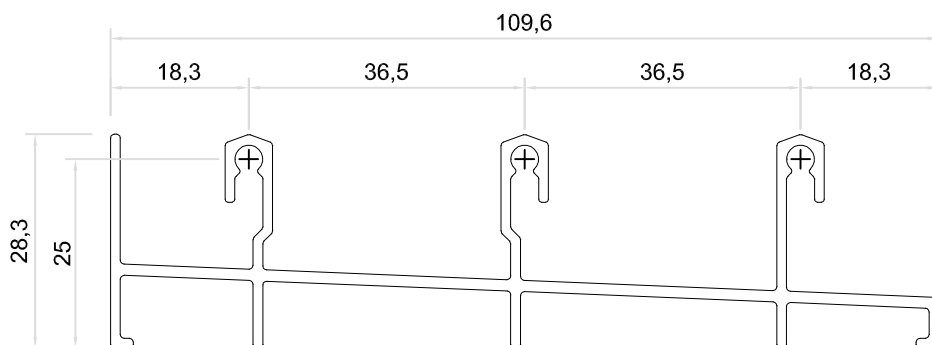
6959 RIEL INFERIOR 3 LINEAS Peso : 0.986 Kg/M Espesor : 1.3 mm Largo : 6,00 mts
