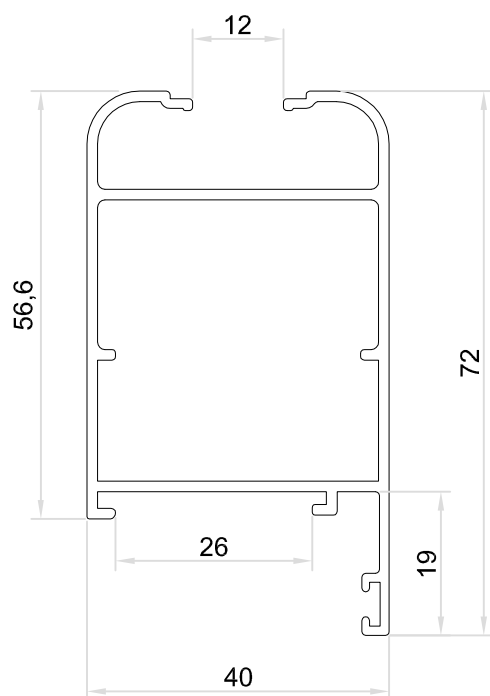
4329 BASTIDOR DE PUERTA LOGGIA Peso : 0.908 Kg/M Espesor : 1.4 mm Largo : 6,00 mts
