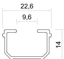
6943 ADAPTADOR MONOLITICO Peso : 0.160 Kg/M Espesor : 1.0 mm Largo : 6,00 mts Color : Negro
