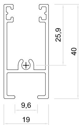
6907 CABEZAL Peso : 0.437 Kg/M Espesor : 1.3 mm Largo : 6,00 mts
