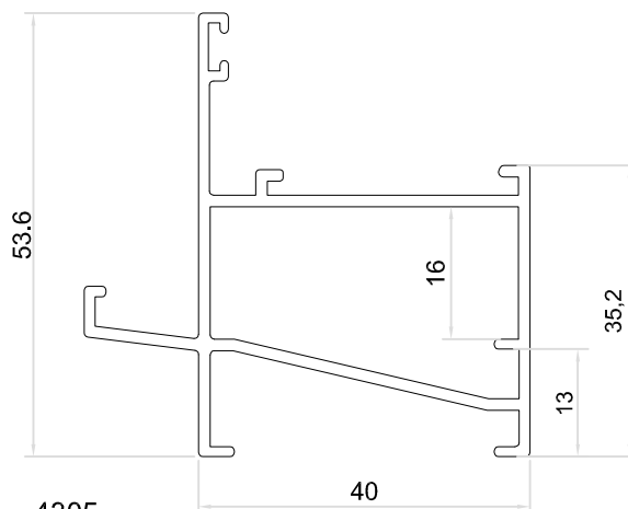
4305 CAMARA DE AGUA EXTERIOR
