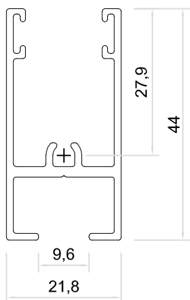
6909 CABEZAL PUERTA VENTANA Peso : 0.520 Kg/M Espesor : 1.3 mm Largo : 6,00 mts
