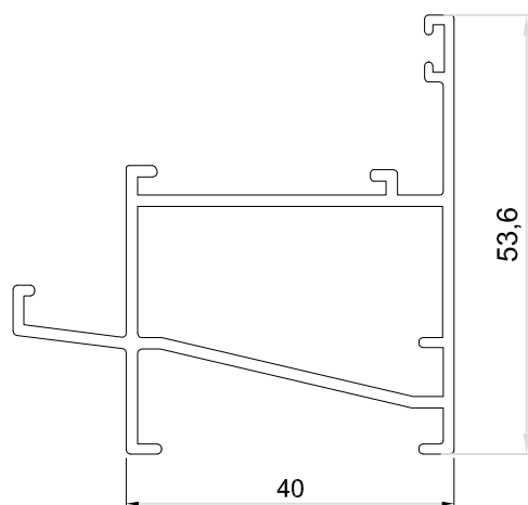
4324 CAMARA DE AGUA INTERIOR Peso : 0.759 Kg/M Espesor : 1.4 mm Largo : 6,00 mts
