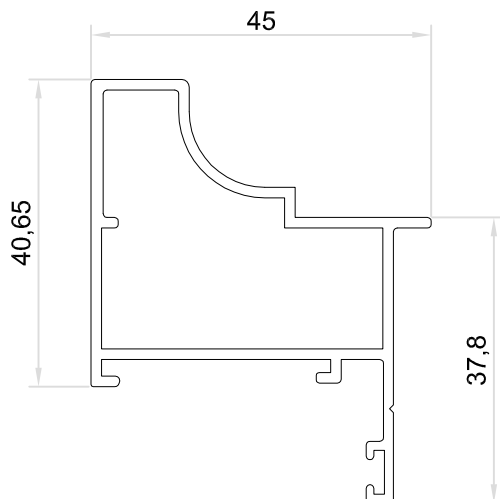
4319 HOJA SILICONA ESTRUCTURAL Peso : 0.706 Kg/M Espesor : 1.4 mm Largo : 6,00 mts
