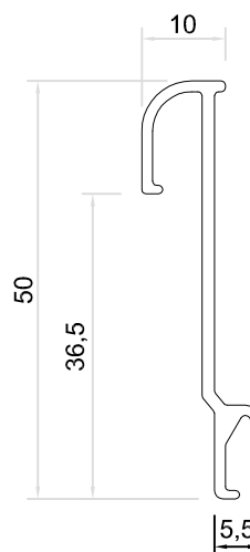
6973 GRADA DE BUQUE Peso : 0.308 Kg/M Espesor : 1.5 mm Largo : 6,00 mts
