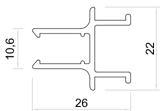
6919 ADAPTADOR CUARTA HOJA Peso : 0.276 Kg/M Espesor : 1.3 mm Largo : 6,00 mts
