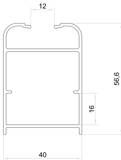
4330 ZOCALO DE PUERTA LOGGIA Peso : 0.808 Kg/M Espesor : 1.4 mm Largo : 6,00 mts
