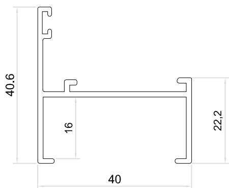
4301 MARCO DOBLE CONTACTO
