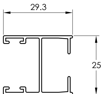
2534 Y PIERNA HOJA FIJA Largo: 6.0 Y 4.85 mt.
