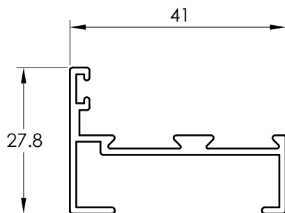
3502 Y MARCO
