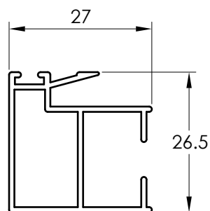
2019 Y TRASLAPO
