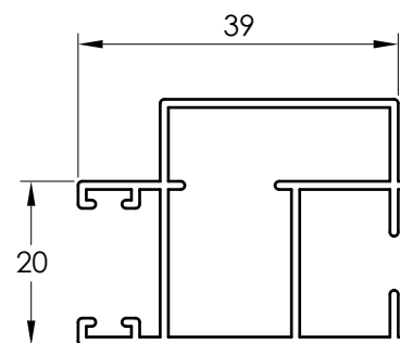
2012 Y PIERNA REFORZADA
