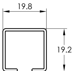
5322 Y RIEL PLUMILLA
