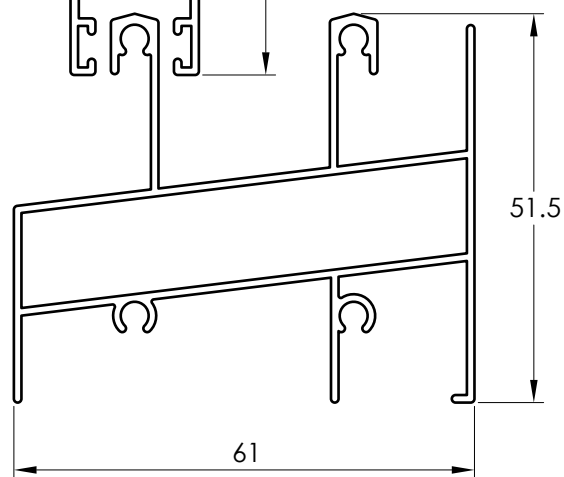
2013 Y RIEL CAMARA DE AGUA
