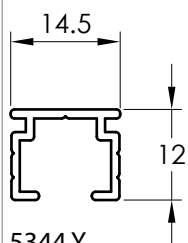
5344 Y RIEL CORTINA
