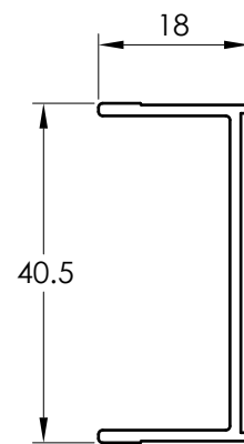
1202 Y JAMBA
