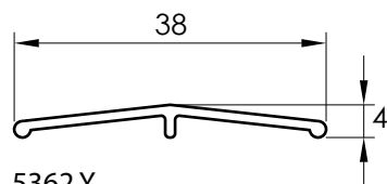
5362 Y CUBREJUNTA
