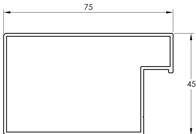
4501 Y BASTIDOR
