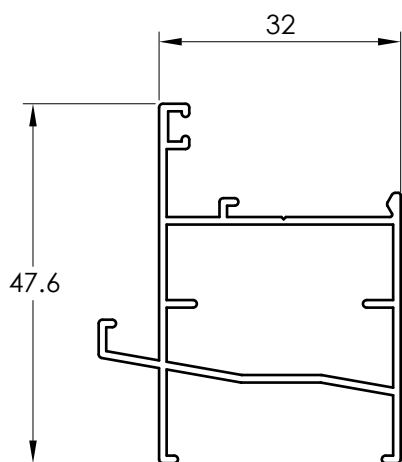
3205 Y MARCO CAMARA DE AGUA
