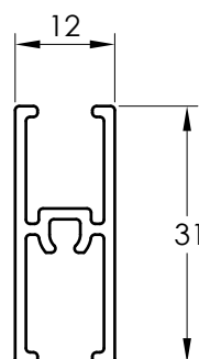
1205 Y PALILLO
