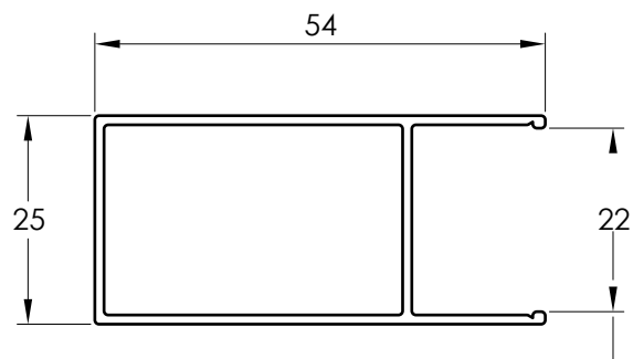
2518 Y PIERNA DOBLE VIDRIO Largo: 6.0 Y 4.85 mt.
