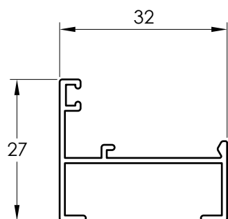
3201 Y MARCO
