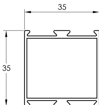
3508 Y BASTIDOR LIVIANO
