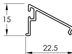
3208 Y JUNQUILLO
