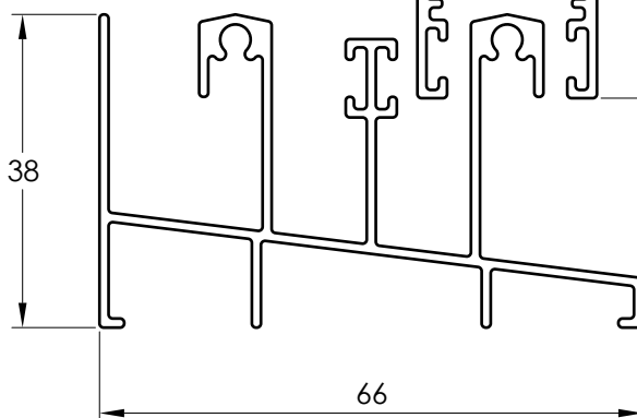
2514 Y RIEL PORTAFELPA
