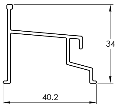
1201 Y RIEL INFERIOR
