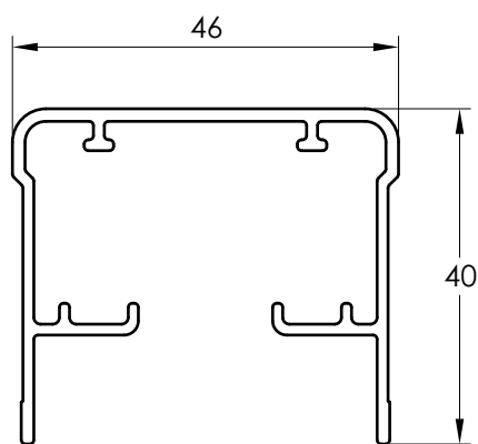
1203 Y RIEL SUPERIOR
