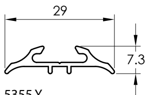
5355 Y CUBREJUNTA
