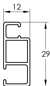
5317 Y MOSQUITERO
