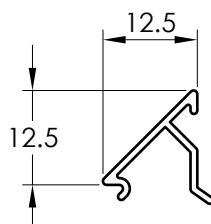
3503 Y JUNQUILLO 45°
