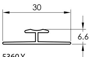
5360 Y TAPA JUNTA
