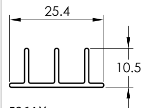
5364 Y DOBLE RIEL
