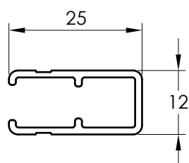
1204 Y BASTIDOR HOJA
