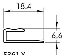
5361 Y TAPA CANTO
