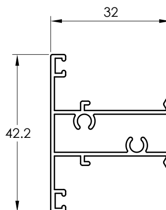
3204 Y PALILLO
