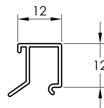
3504 Y JUNQUILLO RECTO
