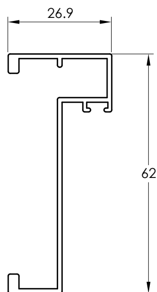
4502 Y MARCO
