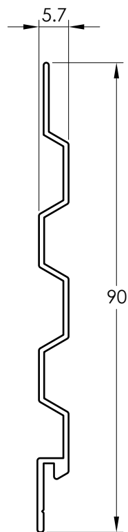
5372 Y RECUBRIMIENTO
