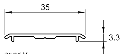
3506 Y TAPA LISA
