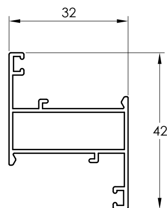
3202 Y HOJA
