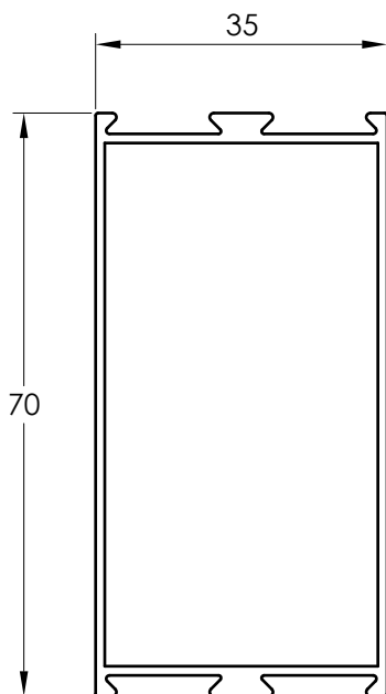
3501 Y BASTIDOR
