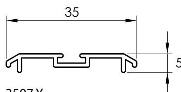
3507 Y TAPA PORTAFELPA
