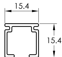
5341 Y RIEL CORTINA
