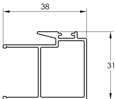
2519 Y TRASLAPO DOBLE VIDRIO Largo: 6.0 Y 4.85 mt.
