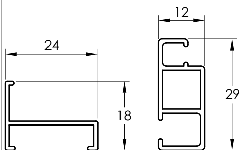
5311 Y MARCO FIJO
