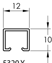
5320 Y JUNQUILLO
