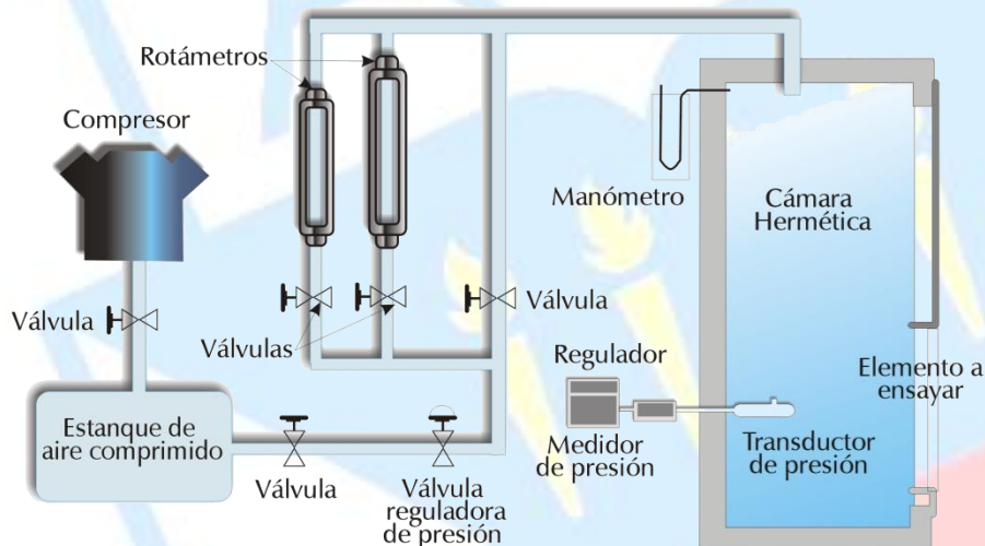
Figura N°1: Esquema montaje experimental
