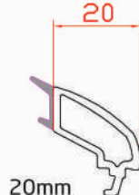
Double Glazing Bead Profile Double Parclose بروفيل نافذة للزجاج المزدوج
