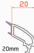
Double Glazing Bead Profile Double Parclose بروفيل نافذة للزجاج المزدوج
