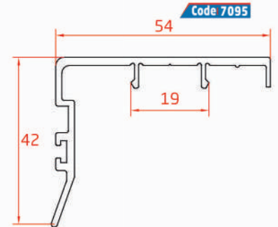
Sliding Sash Closure Profile Ouvrant Couissant Fermeture Profilé بروفيل إغلاق الجناح المنزلق
