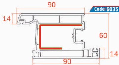
Inside Opening Door Sash Profile Ouvrant à L'ouverture Intérieure "PORTE" بروفيل باب يفتح باتجاه الداخل
