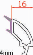
Double Glazing Bead Profile Double Parclose بروفيل نافذة للزجاج المزدوج
