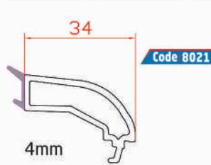
Single Glazing Bead Profile Unique Parclose بروفيل نافذة أحادية الزجاج
