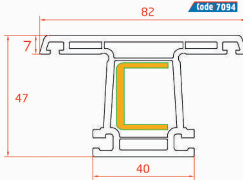
Sliding Mullion Profile Traverse Couissant Profilé بروفيل الإطار المتوسط المنزلق
