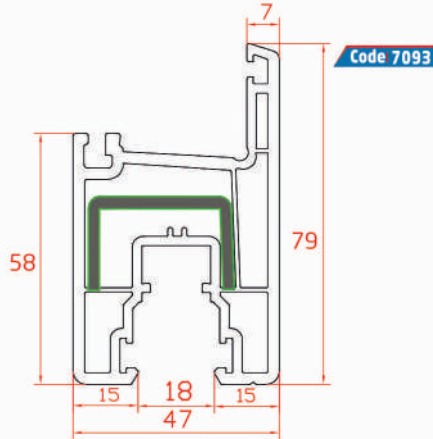
Sliding Sash Profile Ouvrant Couissant Profilé بروفيل الجناح المنزلق
