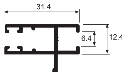
1404 Pierna Reforzada Peso: 0.310 Kg/m Espesor: 1.2 mm
