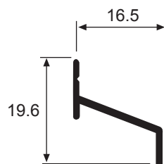
1409 Corta Gotera Peso: 0.105 Kg/m Espesor: 1.2 mm
