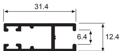
1403 Bastidor Peso: 0.281 Kg/m Espesor: 1.2 mm
