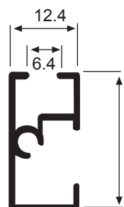
1411 Bastidor Fijo Peso: 0.231 Kg/m Espesor: 1.2 mm
