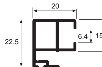
1405 Traslapo Reforzado Peso: 0.300 Kg/m Espesor: 1.2 mm
