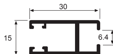
1414 Pierna Corte Recto Peso: 0.290 Kg/m Espesor: 1.2 mm
